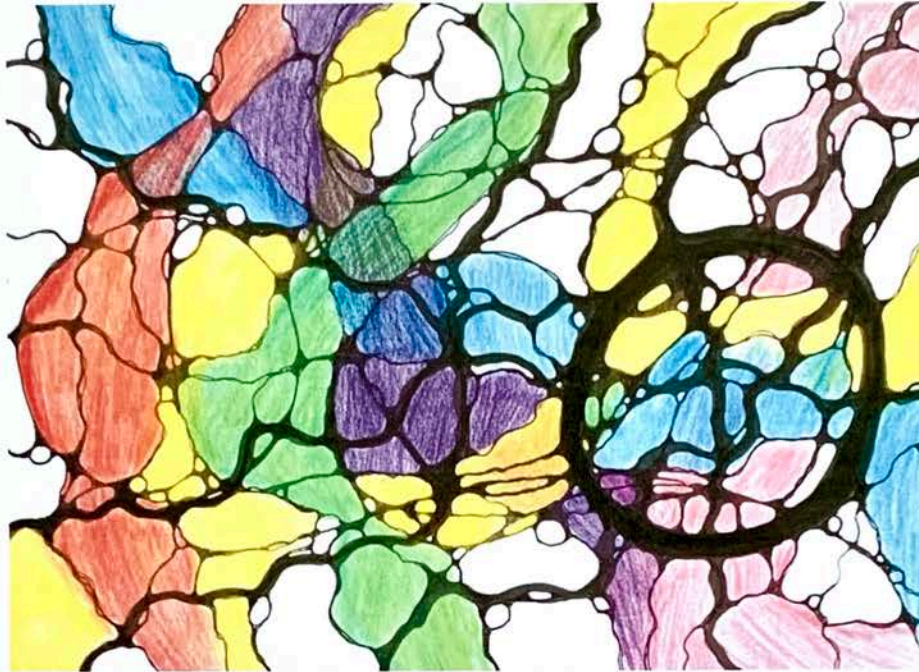
Stephanie Hirmüller
